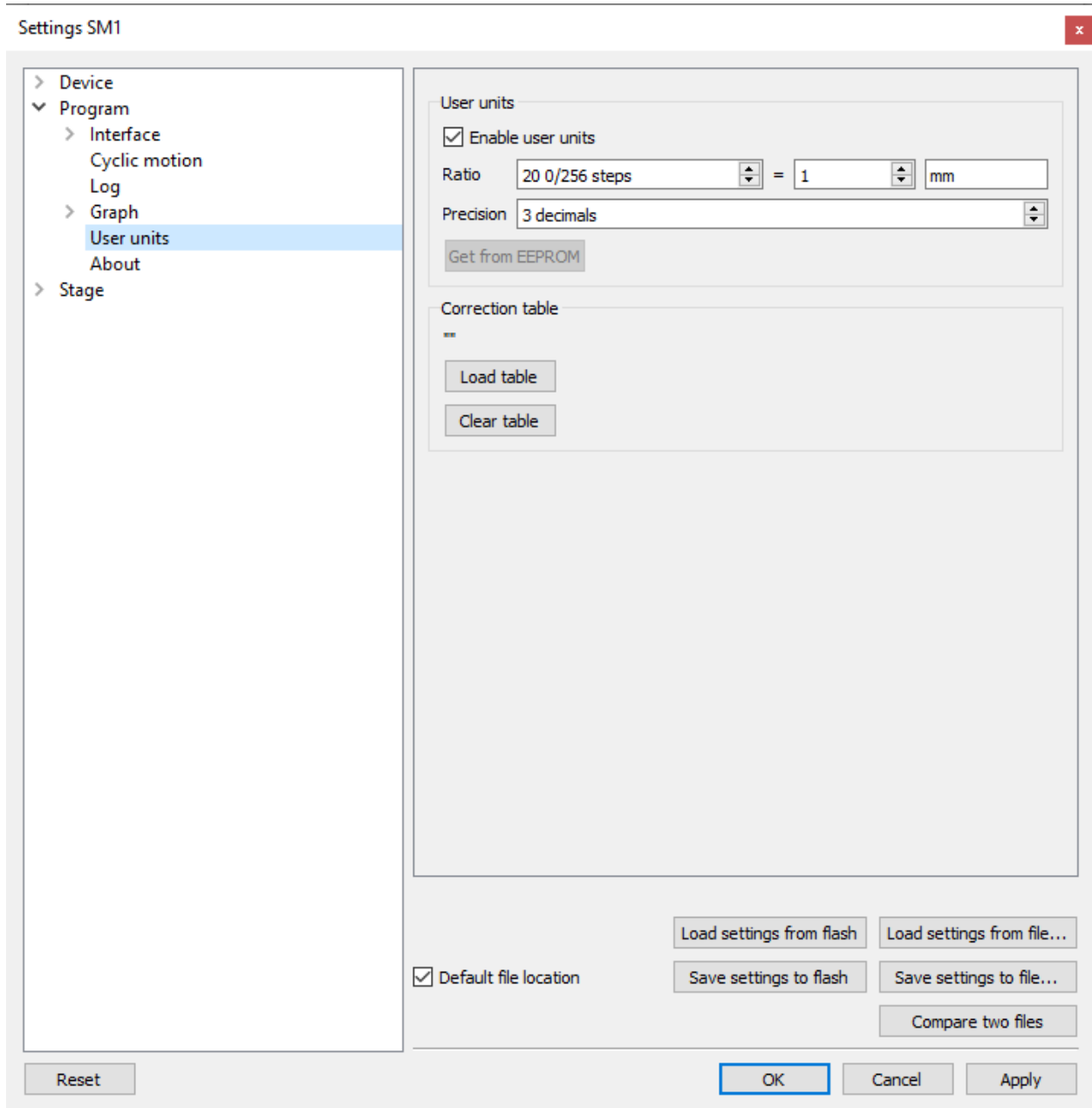
Рис. 5.40: Окно вкладки «Настройки отображения пользовательских единиц»
