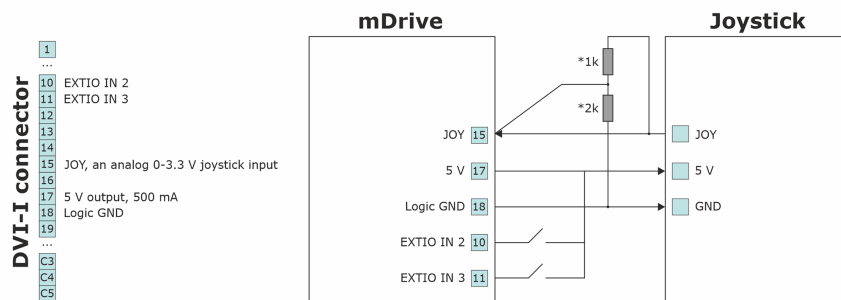
Рис. 4.28: Подключение джойстика (до 5 В) к mDrive через разъем DVI-I (сопротивление «*» рассчитывается индивидуально в зависимости от используемого джойстика)
