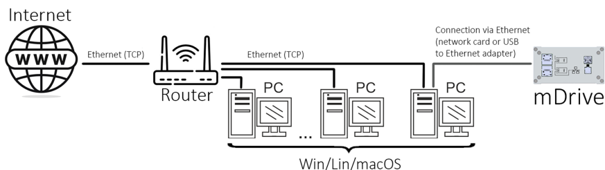
Рис. 7.4: На схеме показано, что, подключив контроллер к компьютеру с помощью кабеля Ethernet или USB - Ethernet адаптера, вы можете найти его в сети и работать с ним. Все компьютеры в сети могут иметь доступ к этому контроллеру.
