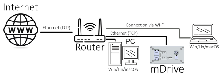
Рис. 7.5: На схеме показано, что, подключив контроллер к локальной сети с помощью кабеля Ethernet, вы можете найти его в сети и работать с ним. Все компьютеры в сети могут иметь доступ к этому контроллеру, включая ноутбуки, подключенные к этой сети через Wi-Fi.
