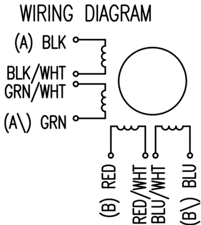
Рис. 3.10: Контакты двигателя
