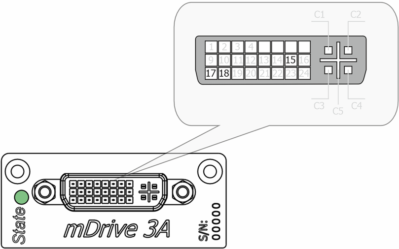
Рис. 4.9: Размеры и нумерация выводов в разъеме DVI-I для подключения джойстика, вид спереди
