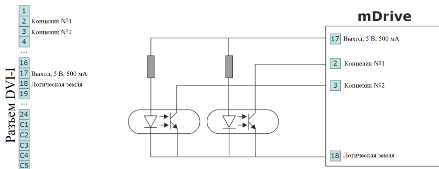
Рис. 4.21: Подключение концевиков типа «оптопара»
