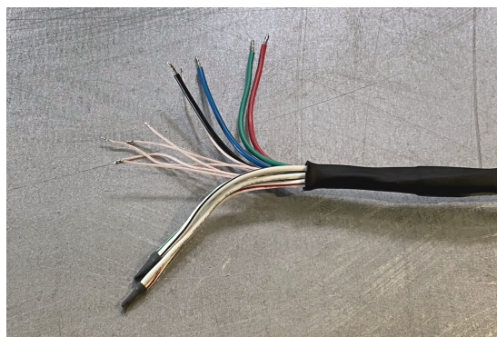
Рис. 3.15: Провода от двигателя и энкодера, собранные при помощи термоусадочной трубки.
