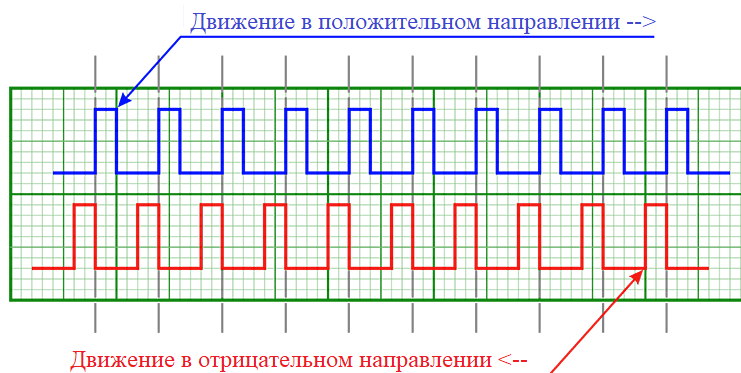
Рис. 4.46: Иллюстрация наложения импульсов синхронизации с заданным шагом соответствующим значению поля «Every» (длительность импульса, измеренная в микросекундах)
