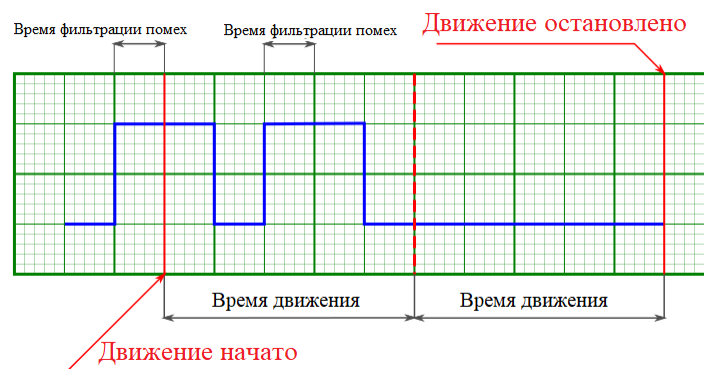
Рис. 4.39: Движение произойдёт один раз на двойное расстояние так как второй импульс синхронизации сработал до окончания первого движения
