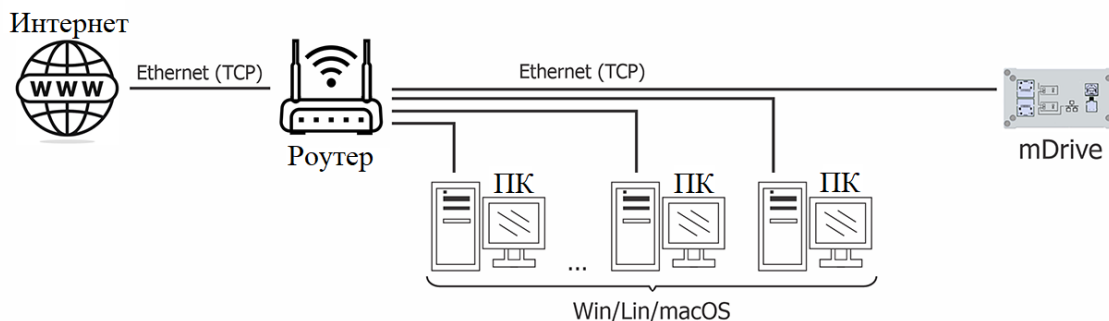
Рис. 7.5: Подключение контроллера mDrive к локальной сети, для обеспечения доступа к управлению из любого ПК сети
