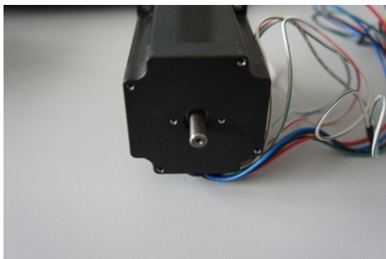
Рис. 3.10: Двигатель без энкодера. Обратите внимание на 2 отверстия M2.5 к которым обычно крепится энкодер
