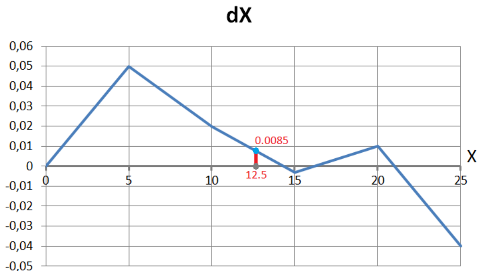
Рис. 4.28: На графике показаны отклонения координат соответствующие таблице
