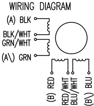
Рис. 3.12: Контакты двигателя
