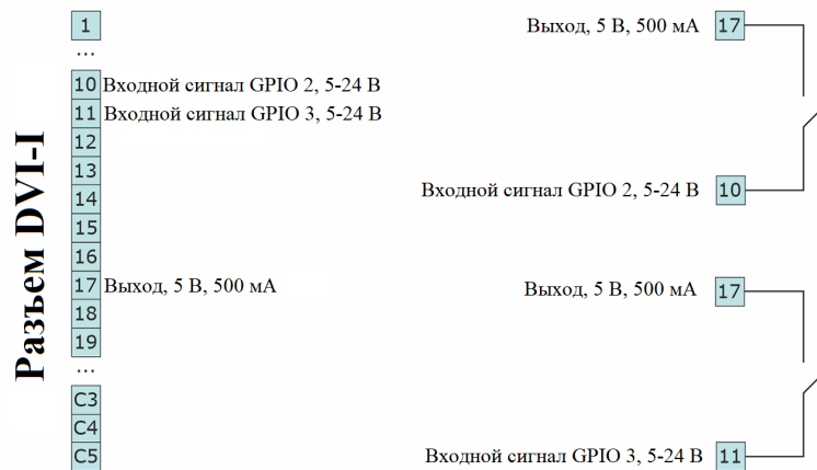
Рис. 4.35: Схема подключения кнопок к разъёму DVI-I к mDrive.
