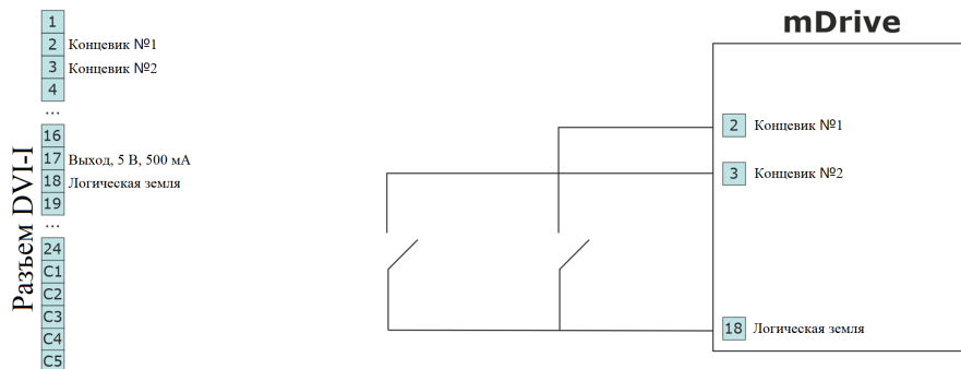
Рис. 4.22: Подключение концевиков типа «сухой контакт»
