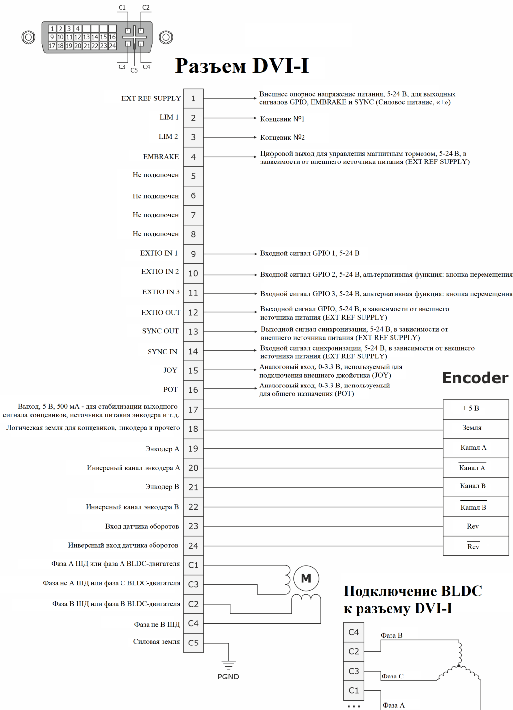
Рис. 3.9: Общая схема подключения позиционера с энкодером через разъем DVI-I
