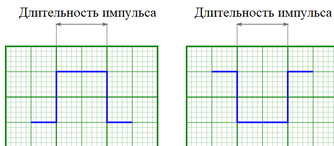
Рис. 4.36: Иллюстрация инвертирования входного или выходного импульса
