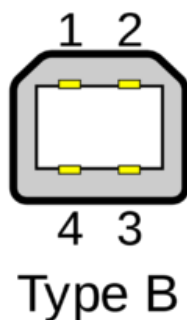
Рис. 4.14: Разъем USB type-B
