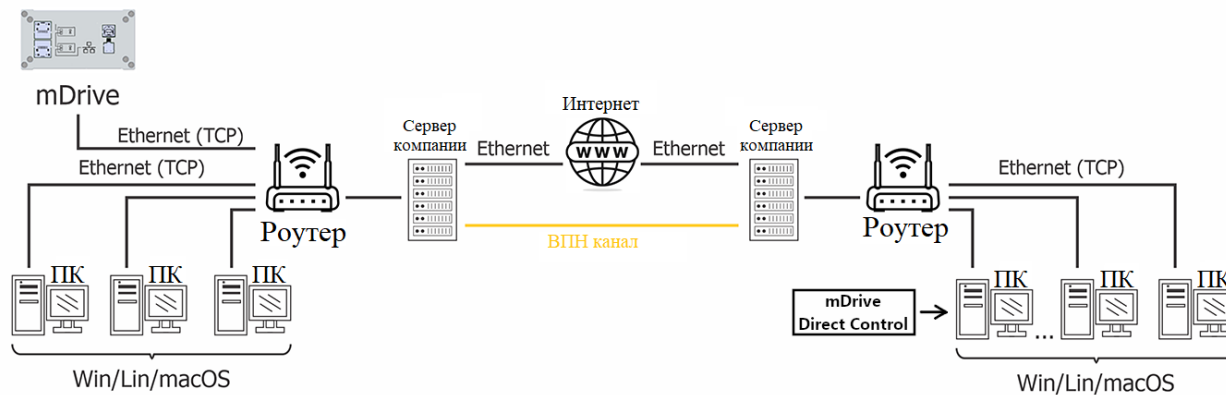
Рис. 7.6: Подключение через VPN к удалённому контроллеру, расположенному в другом офисе
