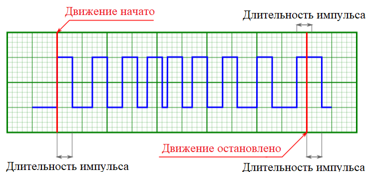
Рис. 4.45: Иллюстрация наложения импульсов синхронизации по старту и по остановке движения, смещение на заданное расстояние (длительность импульса, измеренная в микросекундах)
