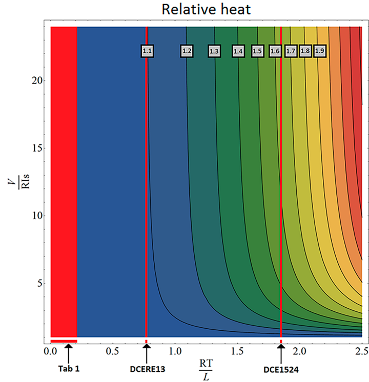
Рис. 4.20: График для оценке перегрева двигателя
