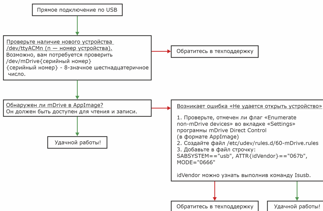
Рис. 8.2: Блок схема диагностики проблем подключения контроллера mDrive через USB (Linux)
