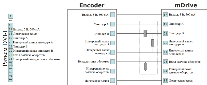
Рис. 4.26: Схема подключения дифференциального энкодера к разъему DVI-I.
