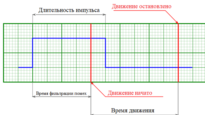
Рис. 4.37: Движение начнётся раз входной импульс дольше времени подавления дребезга
