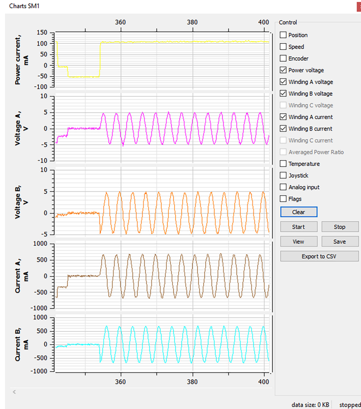
Рис. 8.12: Исправный случай
