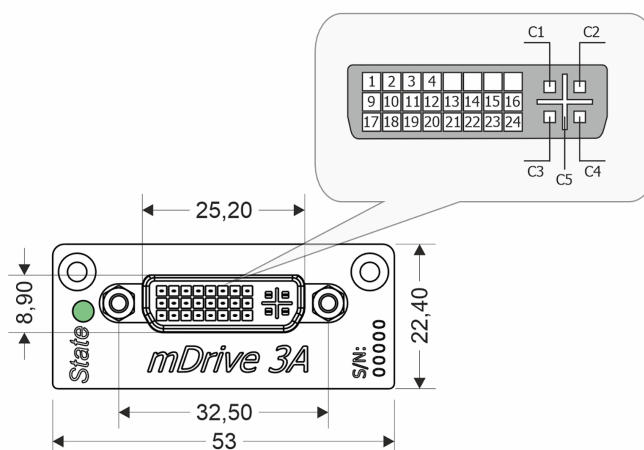
Рис. 4.11: Размеры и нумерация выводов в разъеме DVI-I, вид спереди
