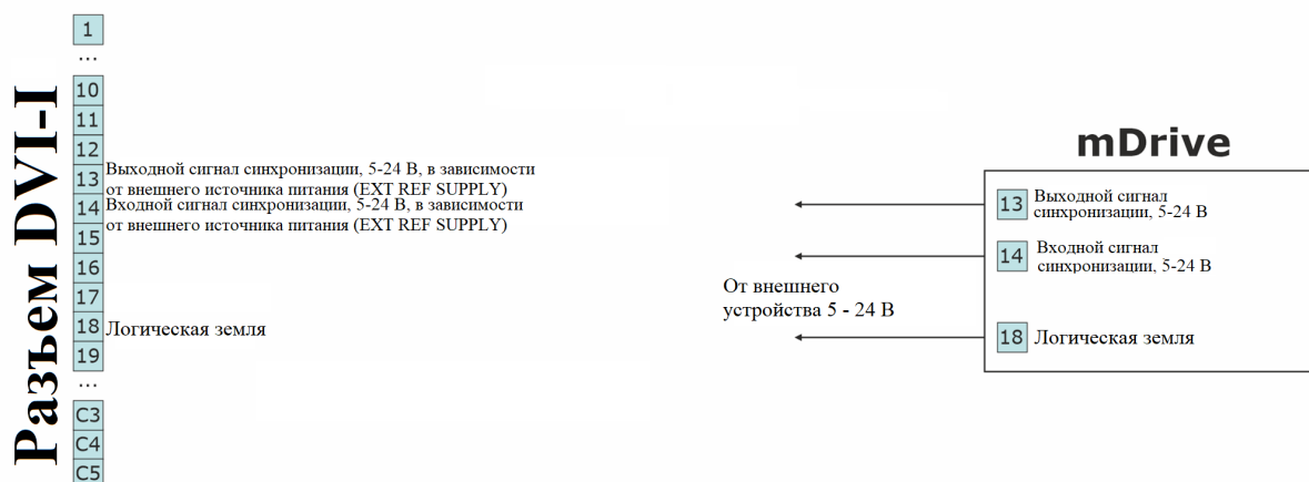
Рис. 4.47: Схема подключения к каналам синхронизации контроллера
