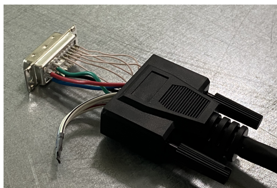
Рис. 3.16: Готовый провод, идущий от двигателя с DVI-I разъёмом на конце
