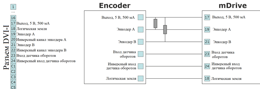
Рис. 4.25: Схема подключения простого энкодера к разъему DVI-I.
