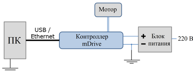
Рис. 2.1: Схема подключения контроллера с заземлением через минусовый провод блока питания
