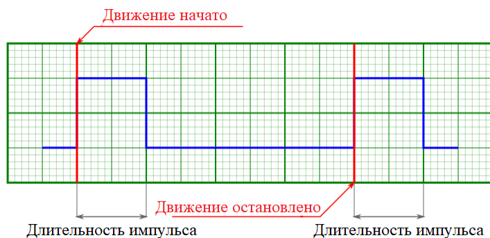
Рис. 4.41: Выходные импульсы синхронизации при генерации их на старте и на остановке движения (импульс фиксированной длительности)
