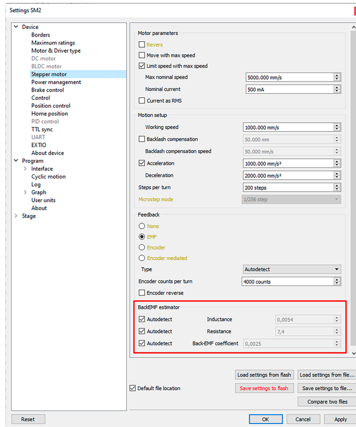
Рис. 4.19: Настройки BackEMF-estimator
