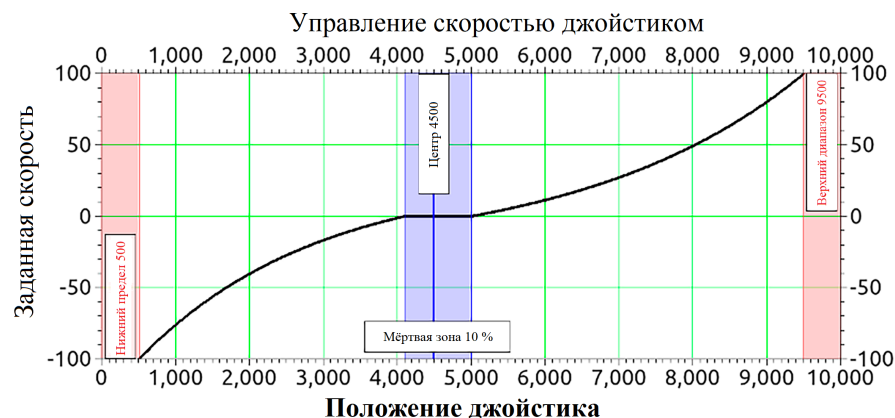
Рис. 4.32: Пример зависимости скорости движения от отклонения джойстика
