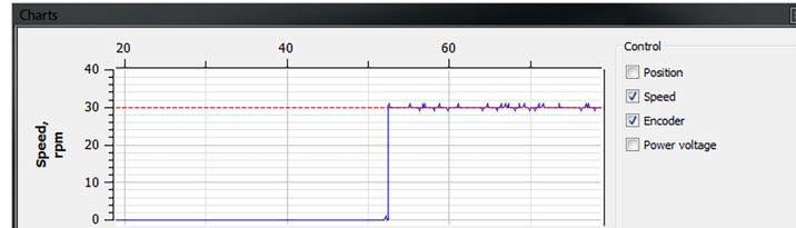
Рис. 5.17: График скорости в программе mDrive Direct Control с ограничением скорости
