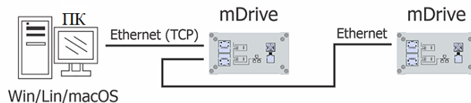
Рис. 7.3: Прямое подключение двух контроллеров mDrive по цепочке к ПК
