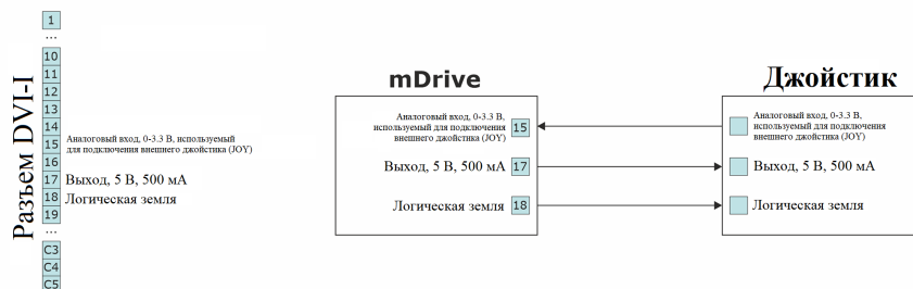
Рис. 4.33: Схема подключения джойстика (до 3.3 В) к mDrive через разъём DVI-I
