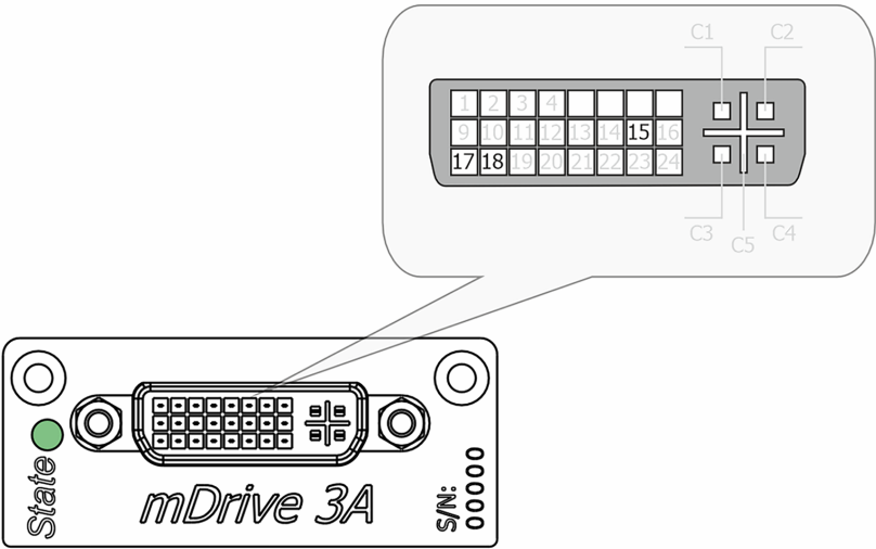
Рис. 4.15: Размеры и нумерация выводов в разъеме DVI-I для подключения джойстика, вид спереди
