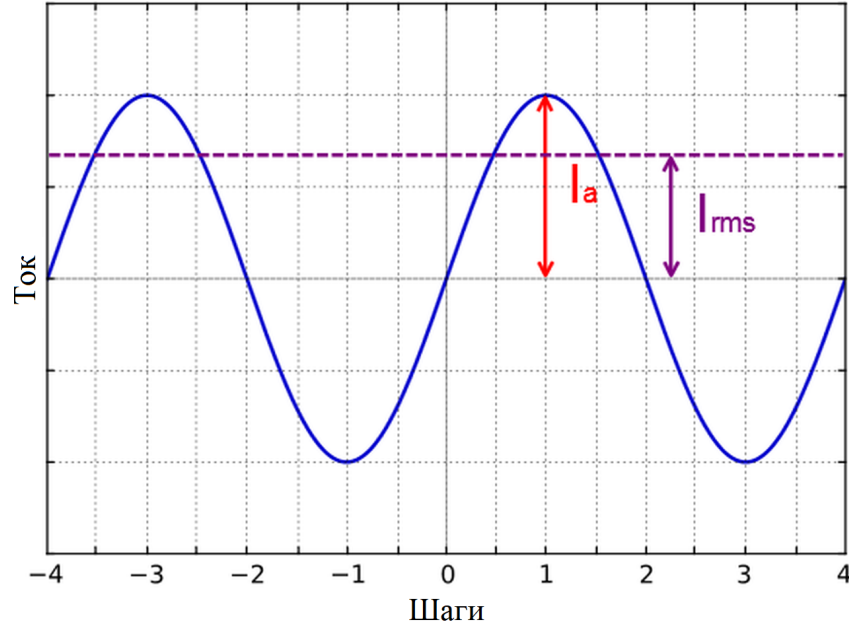
Рис. 3.26: Осциллограмма тока обмотки двигателя и расчёт среднеквадратичного значения
