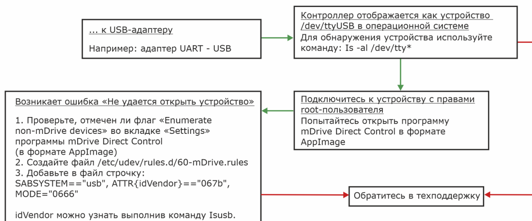
Рис. 8.3: Блок схема диагностики проблем подключения контроллера mDrive через USB-адаптер (Linux)
