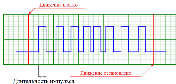
Рис. 4.44: Выходные импульсы синхронизации при движении с ускорением и генерации импульсов каждое смещение на заданное расстояние (импульс измеряется в микросекундах)
