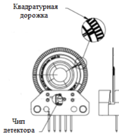
Рис. 4.24: Механика оптического квадратурного энкодера
