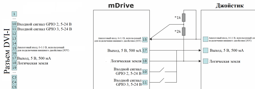
Рис. 4.34: Подключение джойстика (до 5 В) к mDrive через разъем DVI-I (сопротивление «*» рассчитывается индивидуально в зависимости от используемого джойстика)
