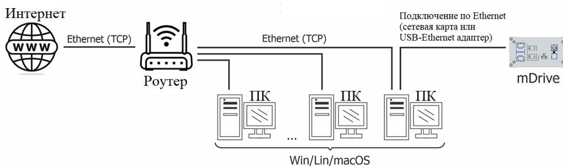
Рис. 7.4: Прямое подключение контроллера mDrive к ПК, подключенному к локальной сети с выходом в сеть Интернет, доступ к управлению ограничен данным ПК
