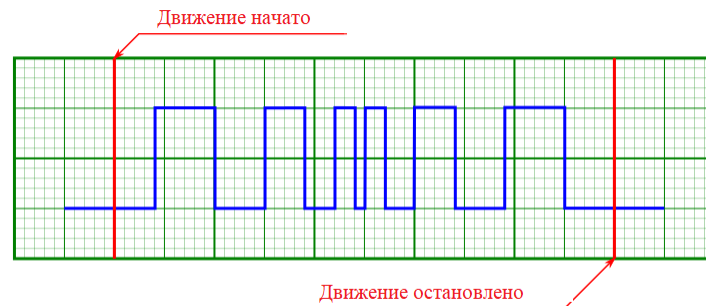
Рис. 4.43: Выходные импульсы синхронизации при движении с ускорением и генерации импульсов каждое смещение на заданное расстояние (импульс измеряется в единицах смещения)
