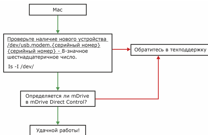
Рис. 8.4: Блок схема диагностики проблем подключения контроллера mDrive через USB (macOS)
