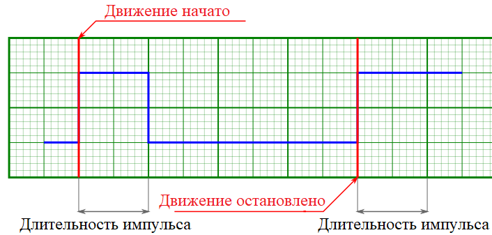
Рис. 4.42: Выходные импульсы синхронизации при генерации их на старте и на остановке движения (импульс измеряется в единицах смещения)
