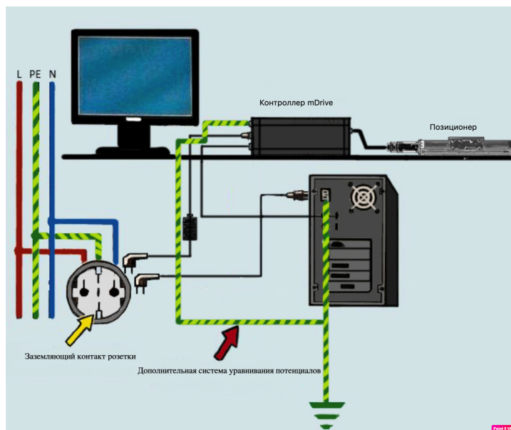
Рис. 8.14: Пример правильного заземления
