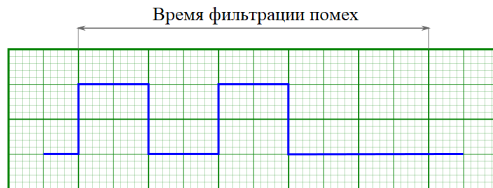
Рис. 4.38: Движение не начнётся так как входные импульсы короче времени подавления дребезга
