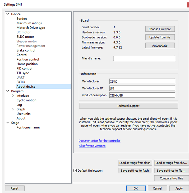
Рис. 5.33: Вкладка «Об устройстве»
