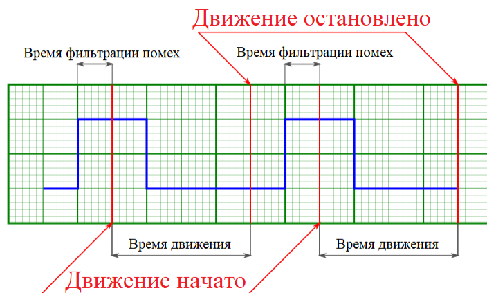
Рис. 4.40: Движение произойдёт два раза с двумя стартами и двумя остановками
