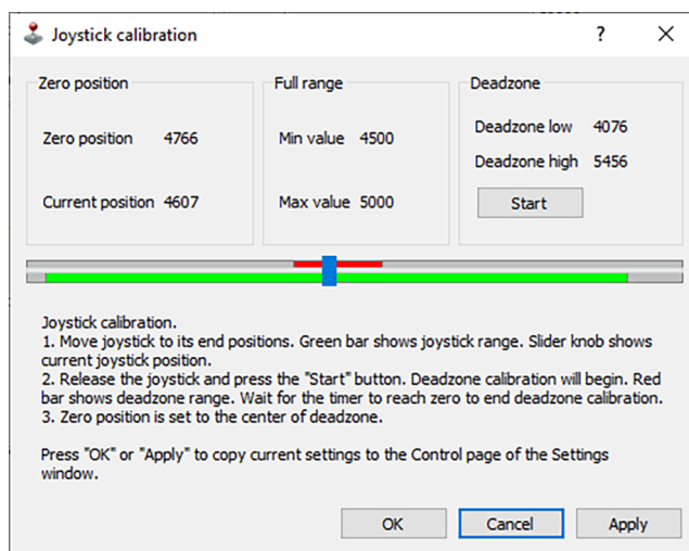
Рис. 5.29: Диалог калибровки джойстика
