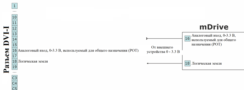
Рис. 4.49: Схема подключения к аналоговому входу в системах mDrive.
