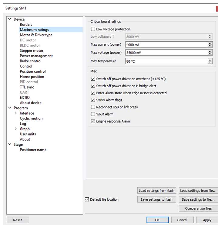
Рис. 5.22: Окно настроек критических параметров контроллера
