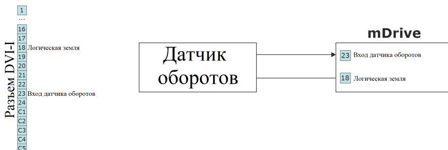
Рис. 4.27: Схема подключения датчика оборотов к системе на базе mDrive
