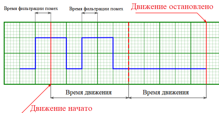
Рис. 4.39: Движение произойдет один раз на двойное расстояние так как второй импульс синхронизации сработал до окончания первого движения
