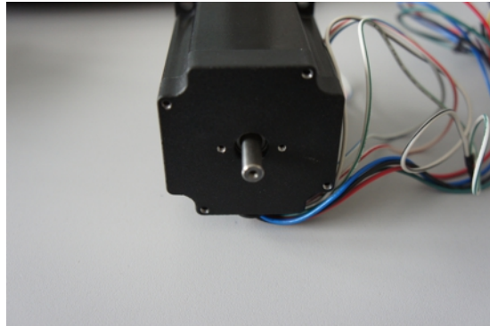
Рис. 3.10: Двигатель без энкодера. Обратите внимание на 2 отверстия М2.5 к которым обычно крепится энкодер
