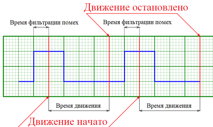
Рис. 4.40: Движение произойдет два раза с двумя стартами и двумя остановками
