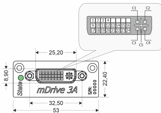
Рис. 4.11: Размеры и нумерация выводов в разьеме DVI-I, вид спереди
