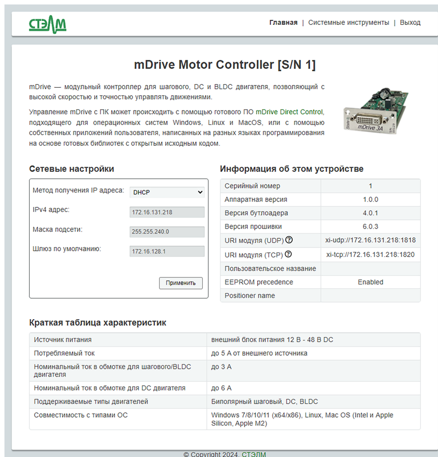
Рис. 8.9: Веб-панель mDrive
