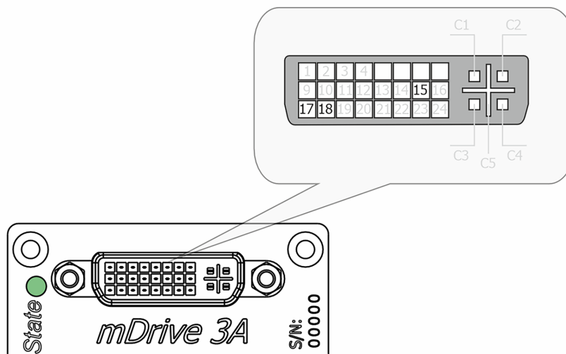
Рис. 4.15: Размеры и нумерация выводов в разьеме DVI-I для подключения джойстика, вид спереди
