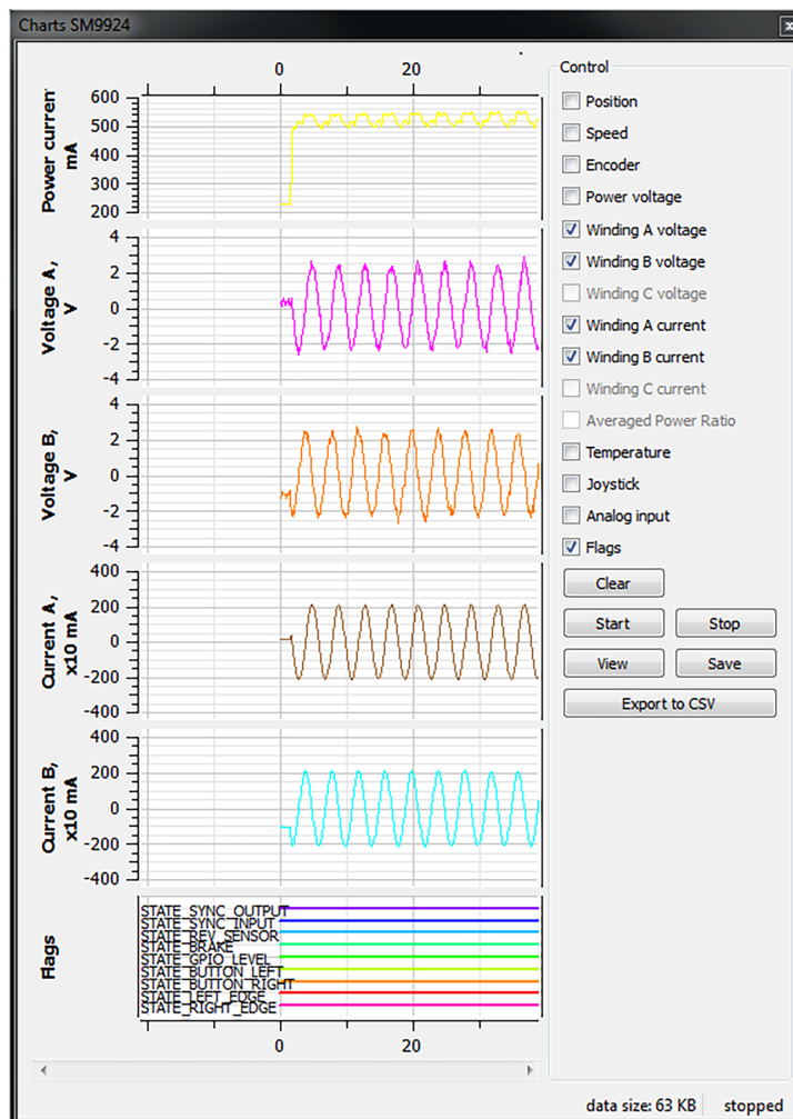
Рис. 5.16: Окно графиков программы mDrive Direct Control
