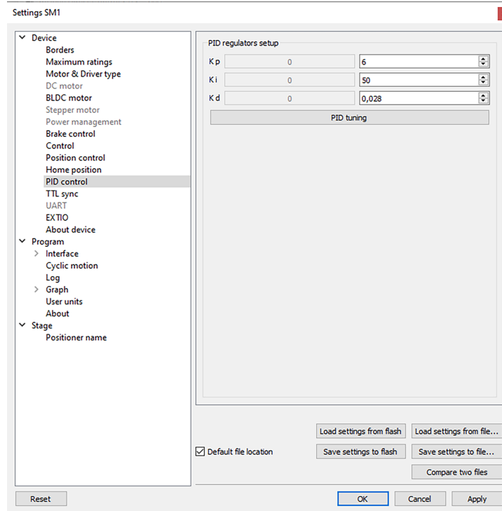
Рис. 5.32: Окно настройки контуров PID-регулирования
