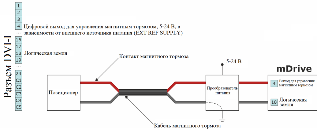
Рис. 4.30: Схема подключения магнитного тормоза к контроллеру mDrive
