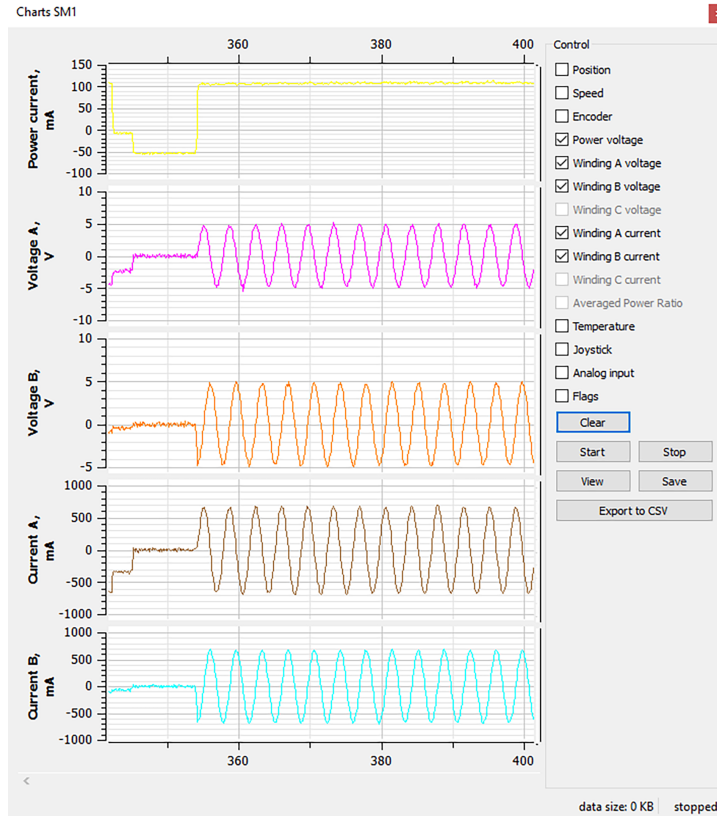
Рис. 8.12: Исправный случай
