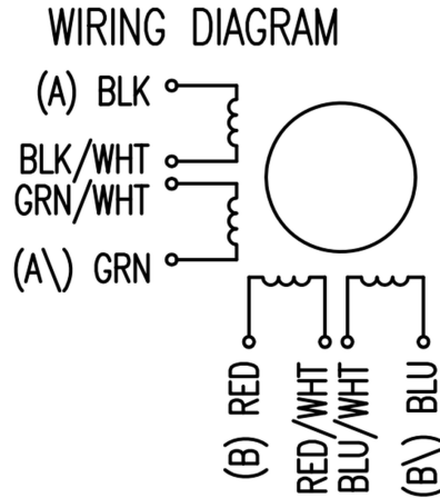
Рис. 3.12: Контакты двигателя
