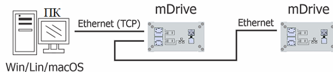
Рис. 7.3: Прямое подключение двух контроллеров mDrive по цепочке к ПК
